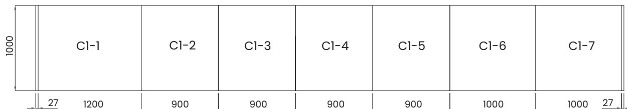
整列柜基础示意
