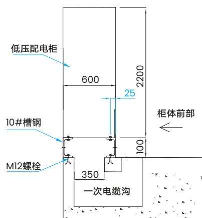
柜体安装示意图(侧视图)
