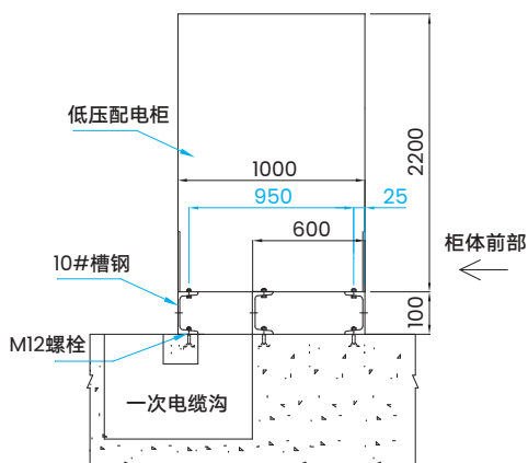
柜体安装示意图(侧视图)
