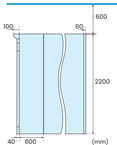
开关柜顶部建议预留空间(侧视图)
