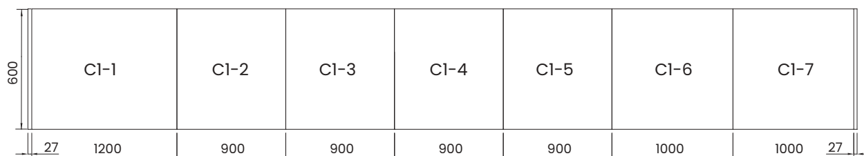
整列柜基础示意
